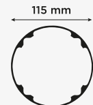
Profil čahure Socket section
