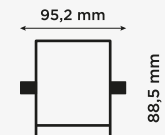
Profil uložka Padding section
