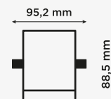
Profil uloška Padding section
