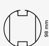
Profil stupa Post section
